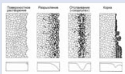
Типовые профили прочности (по Гримму)
